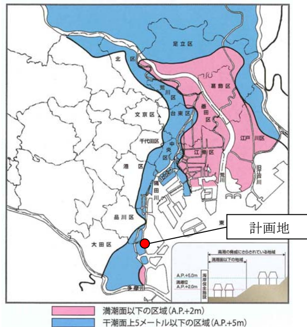
図 9.13-1 東京都区部東部の低地帯
