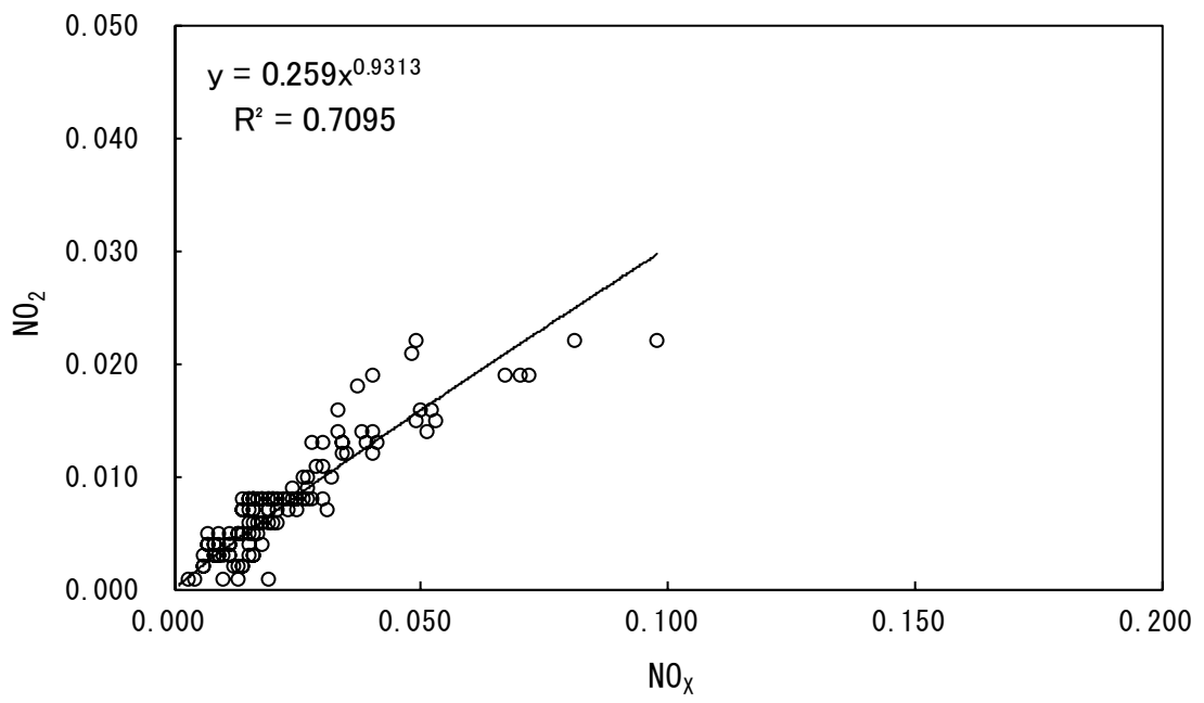
図2.1-5 二酸化窒素 ( \text{NO}_2 ) の変換式の相関図
