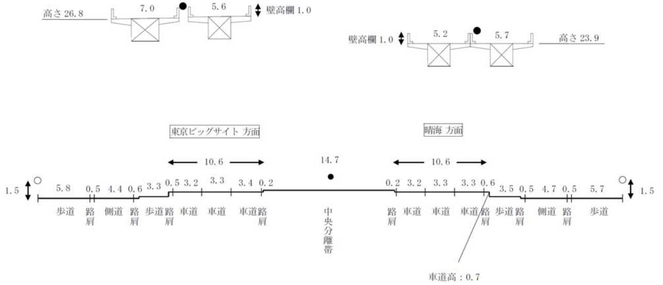
図2.1-4 予測地点の道路断面 (No. 1)
