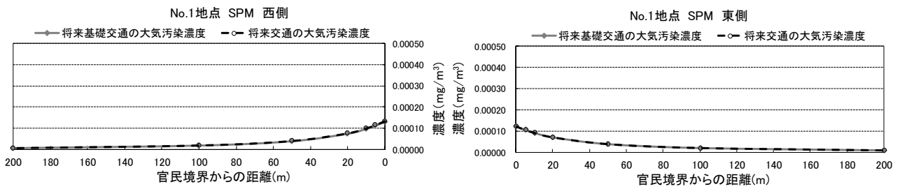
図2.1-6(2) 工事の施行中における浮遊粒子状物質寄与濃度の距離減衰 (No. 1)
